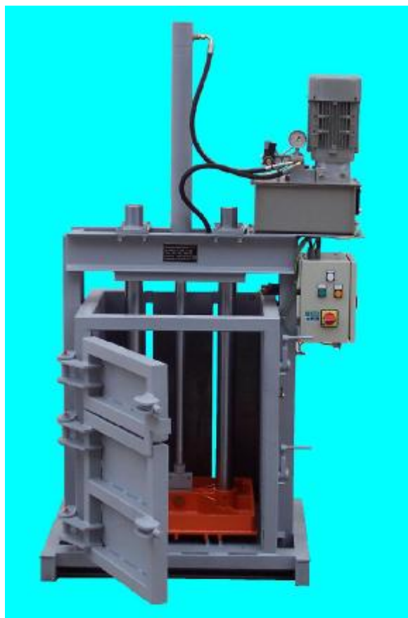
Paketovací lis HPL 6,3 upravený pro lisování plechovek
